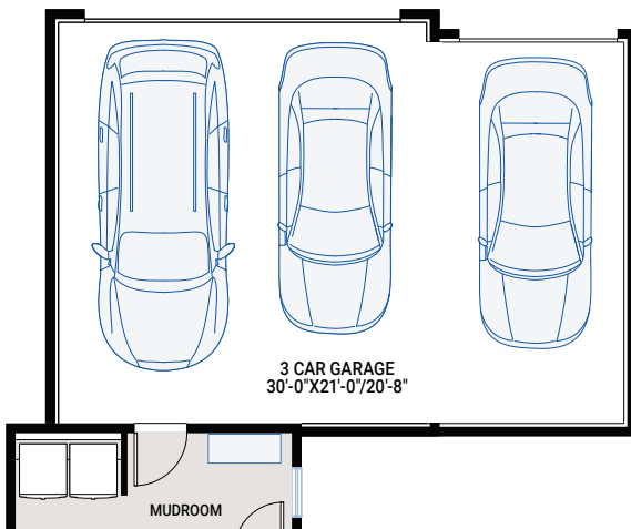
OPTION #05A Optional 3-Car Garage - adds 207 sq ft
