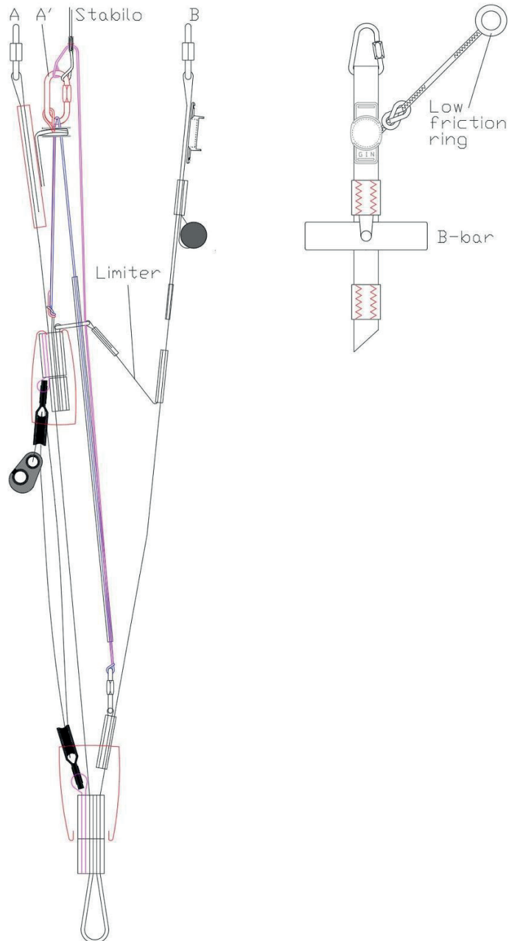
Abbildung: Leopard Tragegurt
