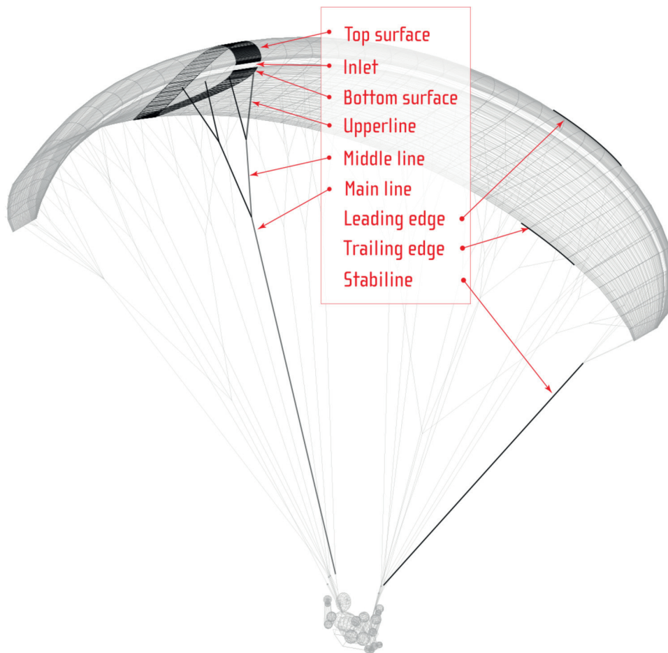
Abbildung: Allgemeine Übersichtszeichnung und Beschreibung der Fallschirmbauteile
