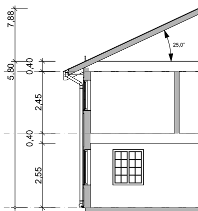
Snitt
