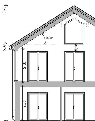
Snitt A
