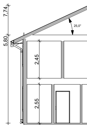
Snitt A
