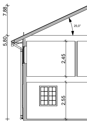
Snitt A
