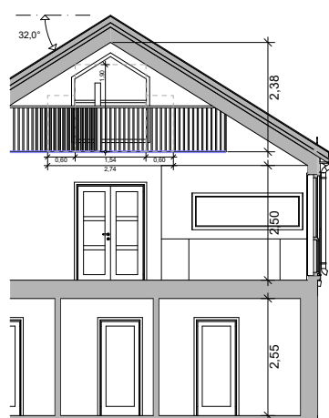
Snitt B
