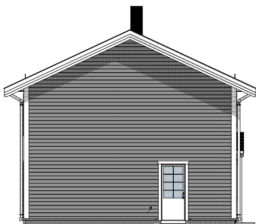
Fasade Øst
