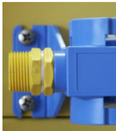
5. Gelben Zulaufstutzen bis zum Anschlag eindrehen
