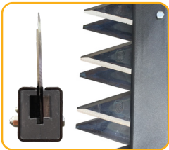
Bilama / Guide PVC - Double blade / PVC support Double section / PVC lamier - Doppelklingen- / PVC-Führungen
