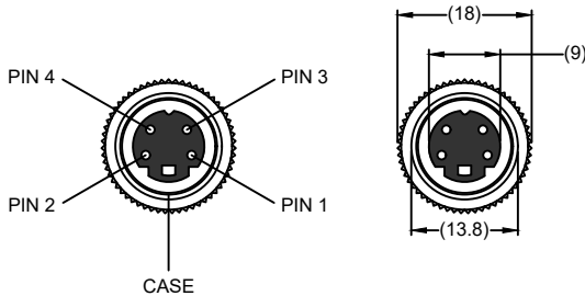
4 PIN MINI DIN FEMALE MATING FACE
