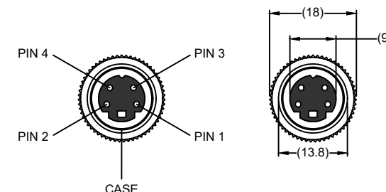
4 PIN MINI DIN FEMALE MATING FACE
