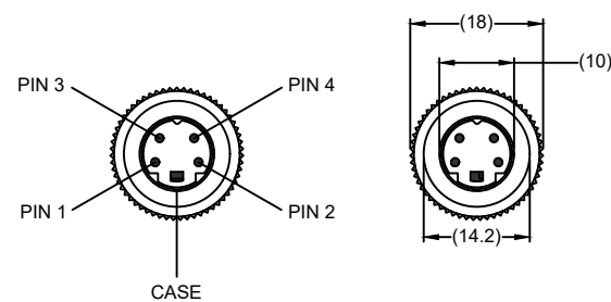
4 PIN MINI DIN MALE MATING FACE
