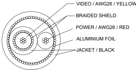
VIEW A-A
