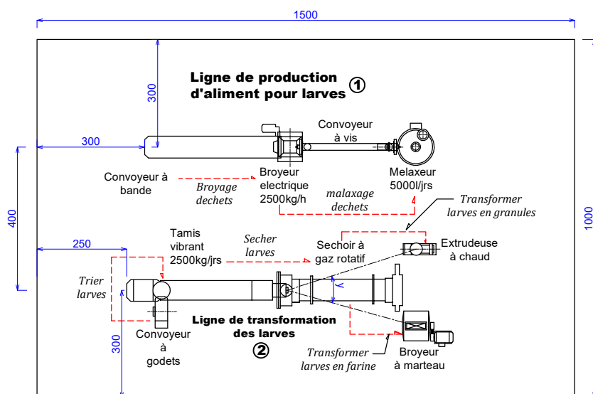
VUE EN PLAN DE L'USINE
